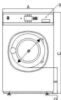
Μπροστινή πλευρά
